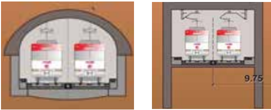
Túnel en mina. Sistema de pantallas.
